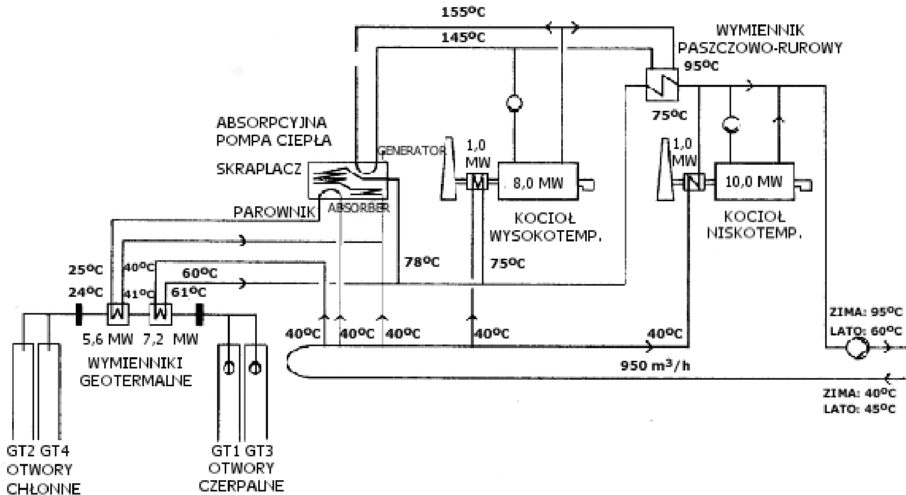
Schemat ideowy ciepłowni geotermalnej w Pyrzycach ( www.inet.com.pl/geotermia/strona002.htm )
